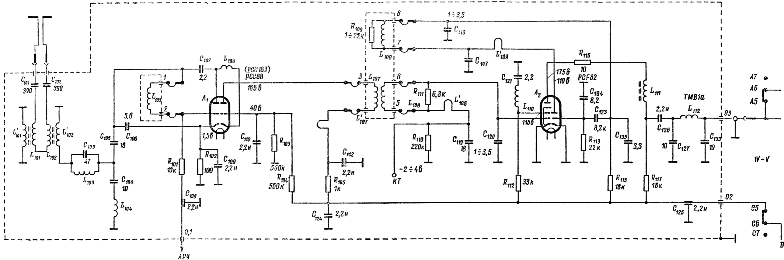
Фиг. 152. Най-често срещана схема на канален превключвател
